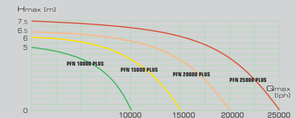
Соотношение производительности помпы и максимальной высоты подъема воды Débit de la pompe par rapport à l'hauteur de levage de l'eau
